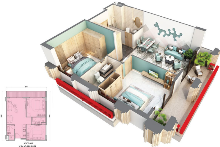
K503-01 CĂN HỘ 2PN SUITE DIỆN TÍCH 75.202
